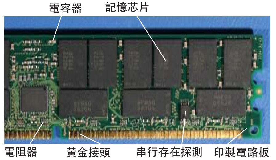
記憶模塊的共同組成零件.
