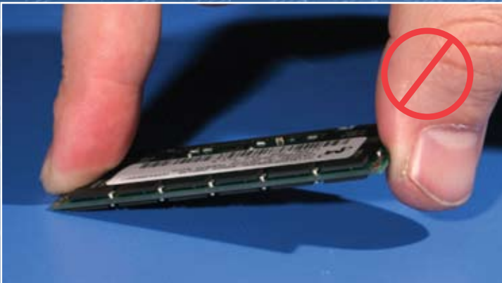
絕不按壓模塊的一側然後向上拔起.
